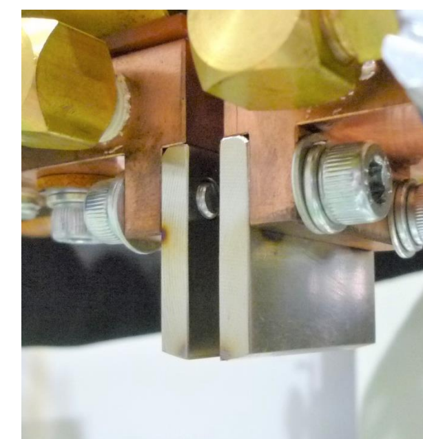
平行電極 Parallel electrode
