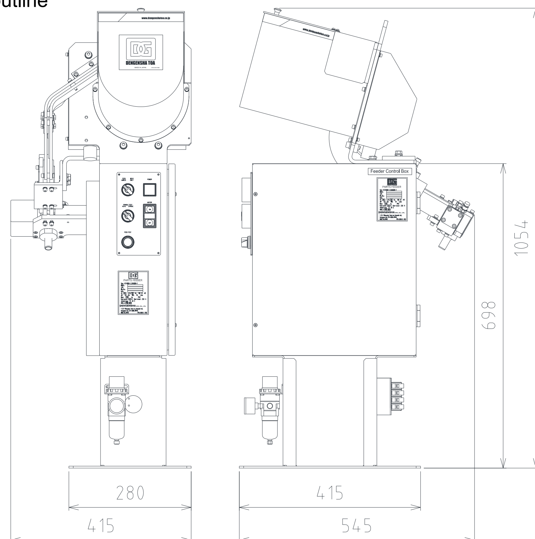
外形図 outline
