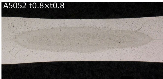
第1通電後に鍛圧・後熱を入れることで クラック・ブローホールを抑制 Cracks and blowholes are suppressed by applying forging force and post- heat after the first current.
